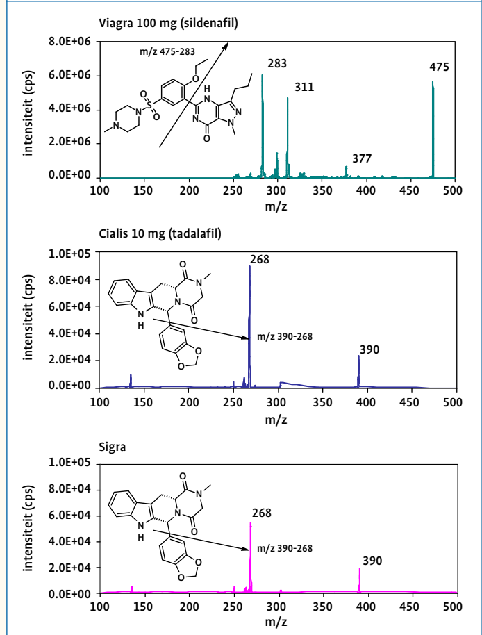
Figuur 1 Massaspectra van Viagra, Cialis en Siga
